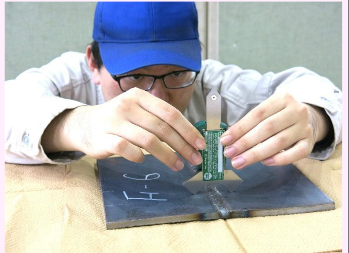
外観試験
