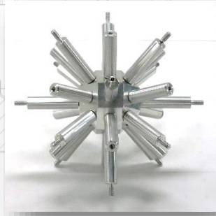
中心部構造 材質：A5052 (旋盤・フライス盤加工)
